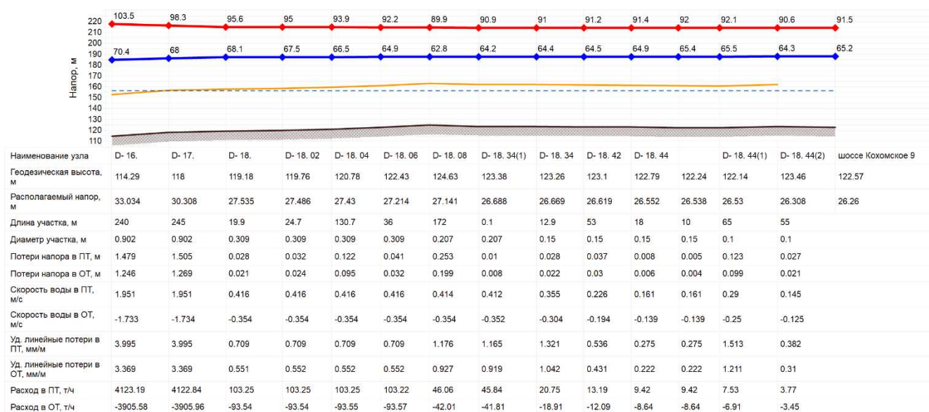
Рисунок 12.1.3.2 Параметры работы теплосети от ИвТЭЦ-3 (вывод D) до ж/д по Кохомскому ш., д.9
