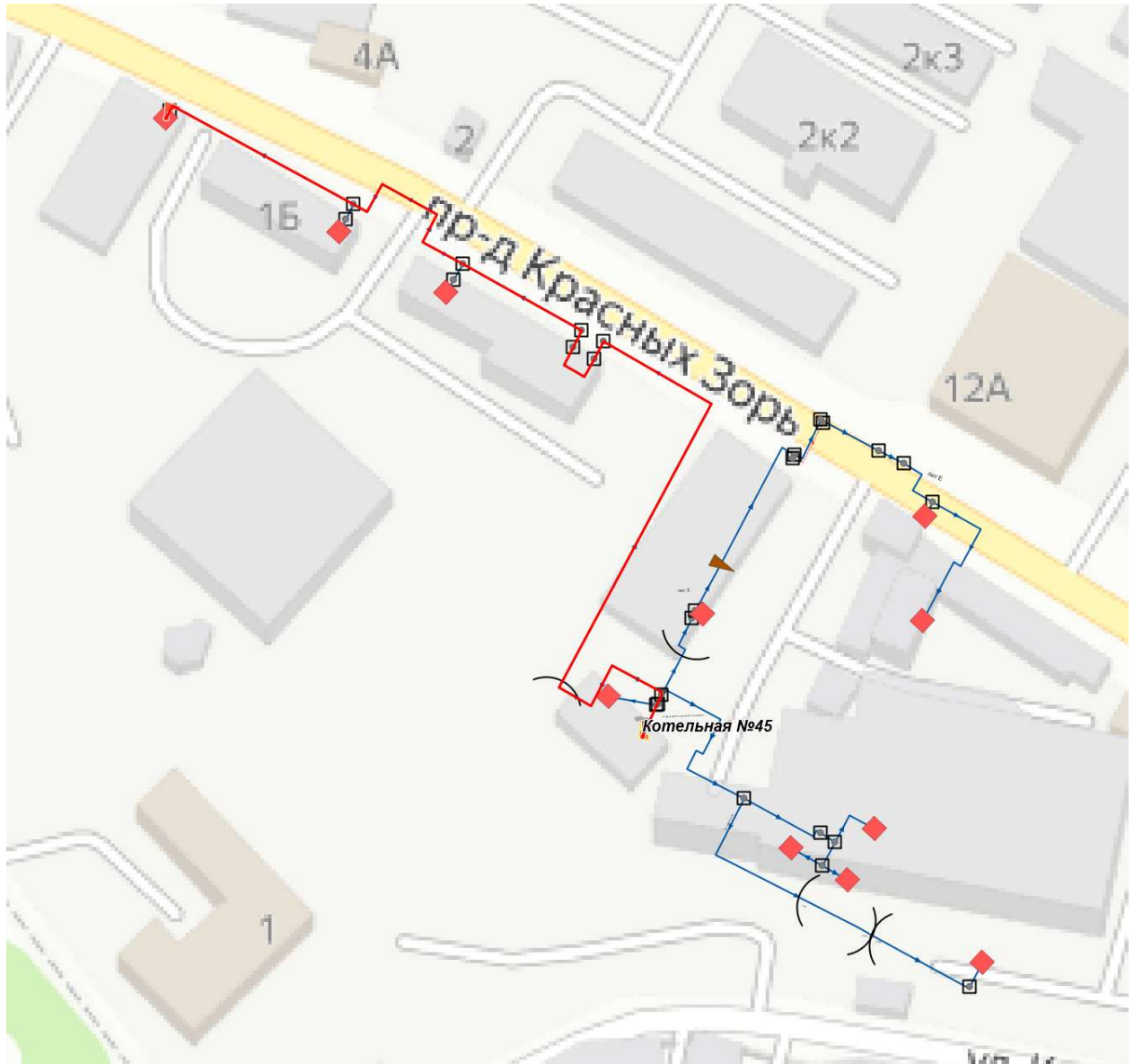
Рисунок 12.2.10.1 Расчетная схема участка теплосети от Котельной №45 до ж/д №16 по проезду Красных Зорь
