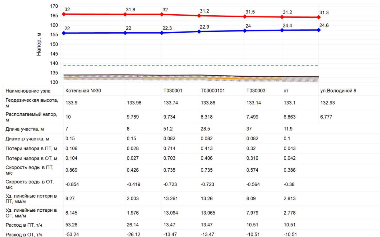
Рисунок 12.2.4.2 Параметры работы теплосети от Котельной №30 до ж/д №9 по ул. Володиной
