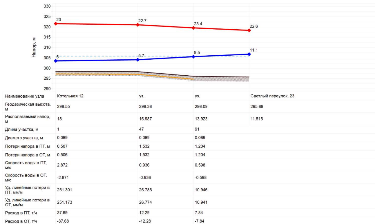
Рисунок 12.2.10.2 Параметры работы теплосети от Котельной №45 до ж/д №16 по проезду Красных Зорь
