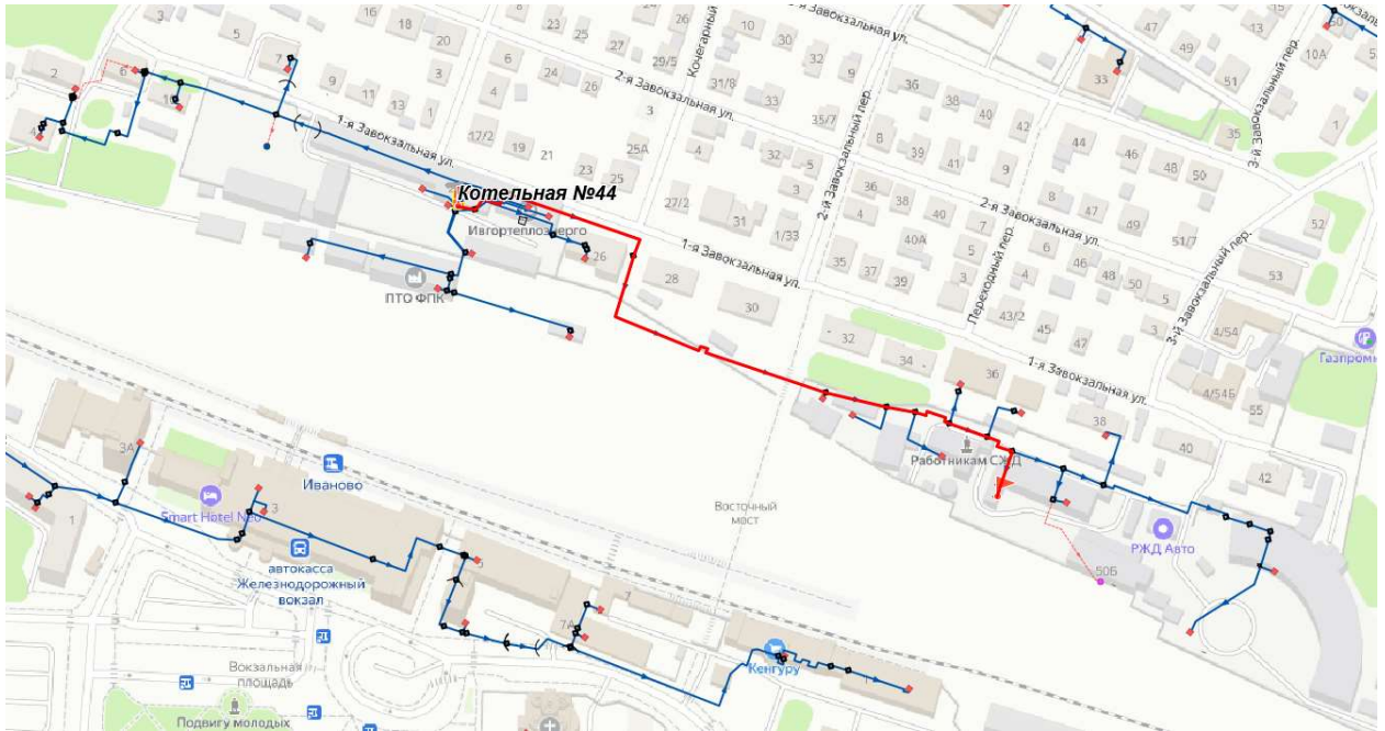
Рисунок 12.2.9.1 Расчетная схема участка теплосети от Котельной №44 до ж/д №50а по ул. 1-я Завокзальная
