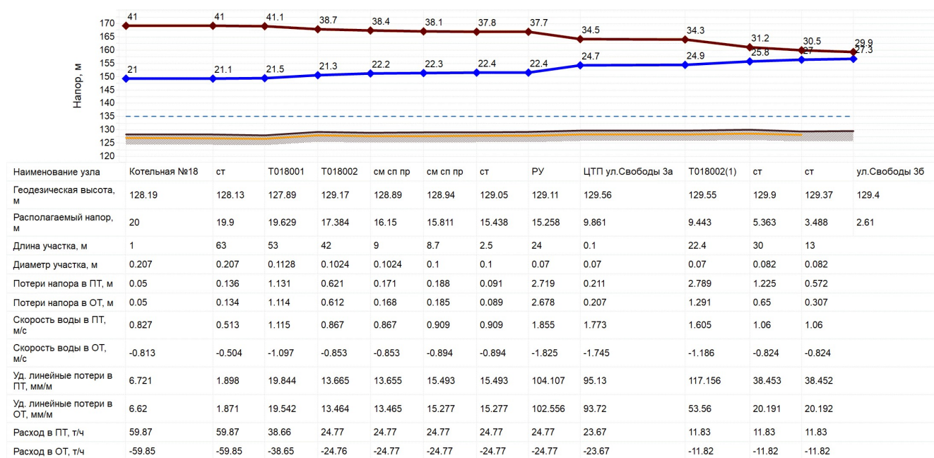
Рисунок 12.2.3.2 Параметры работы теплосети от Котельной №18 до ж/д №36 по ул. Свободы.
