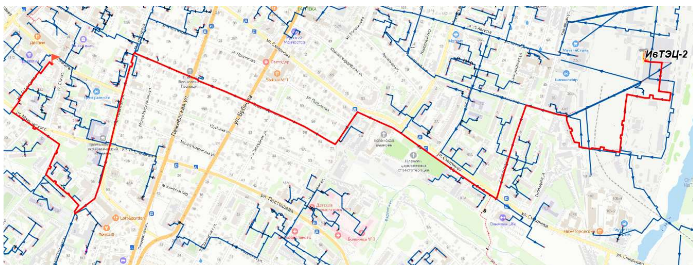
Рисунок 12.1.3.1 Расчетная схема участка теплосети от ИвТЭЦ-2 (вывод С) до ж/д по ул. Багаева, д.11
