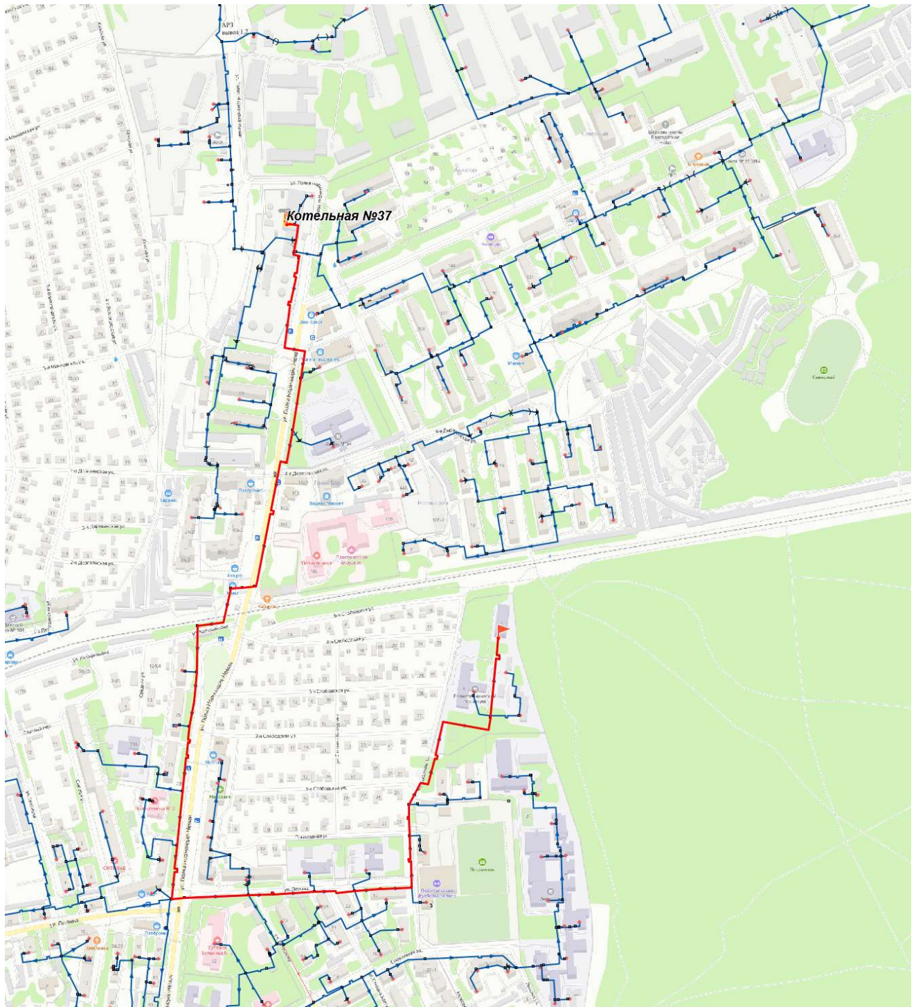
Рисунок 12.2.5.1 Расчетная схема участка теплосети от Котельной №37 до ж/д №4 по ул. Музыкальная
