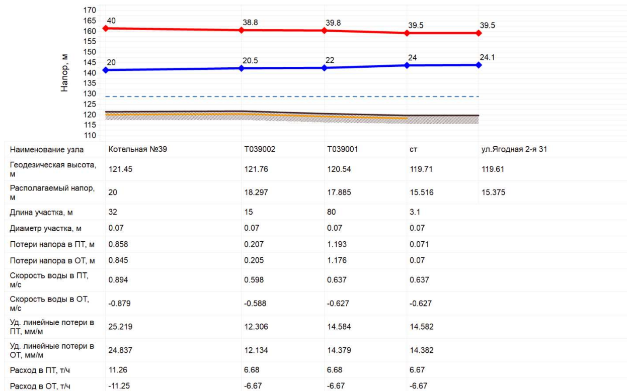
Рисунок 12.2.6.2 Параметры работы теплосети от Котельной №39 до ж/д №31 по ул. 2-я Ягодная
