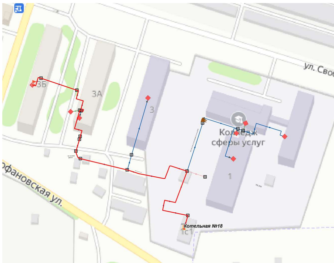
Рисунок 12.2.3.1 Расчетная схема участка теплосети от котельной Котельной №18 до ж/д №36 по ул. Свободы
