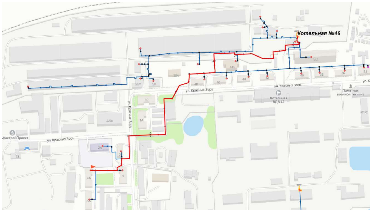
Рисунок 12.2.11.1 Расчетная схема участка теплосети от Котельной №46 до ж/д №4а по ул. Суздальская
