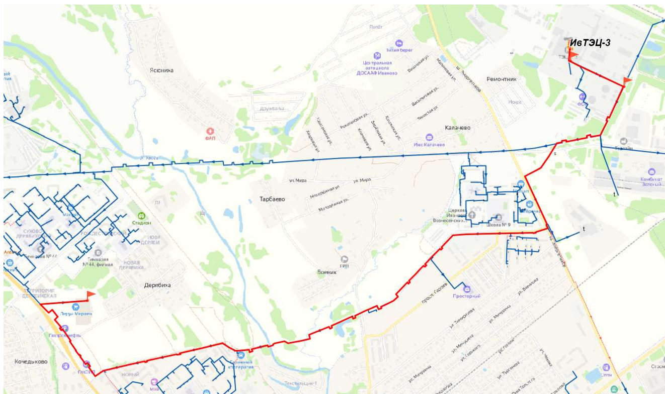
Рисунок 12.1.3.1 Расчетная схема участка теплосети от ИвТЭЦ-3 (вывод Е) до д. Дерябиха
