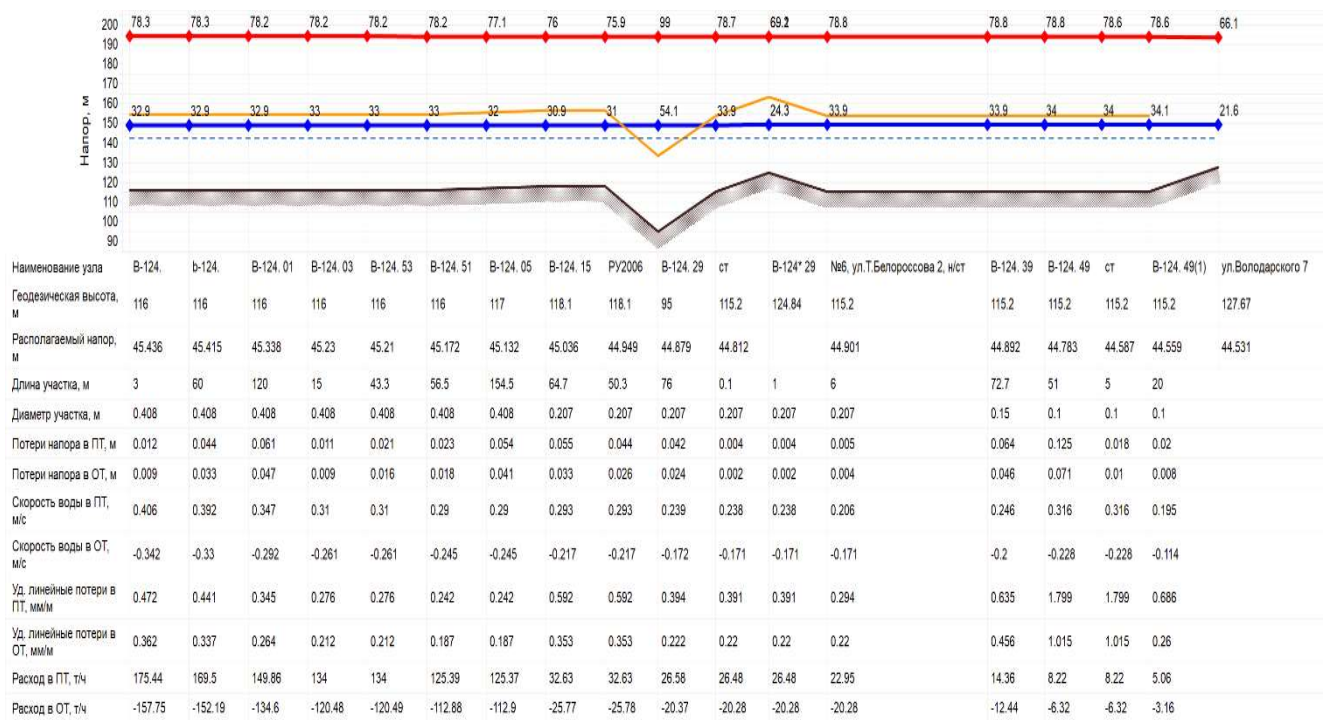
Рисунок 12.1.2.2 Параметры работы теплосети от ИвТЭЦ-2 (вывод В) до ж/д по ул. Володарского, д.7
