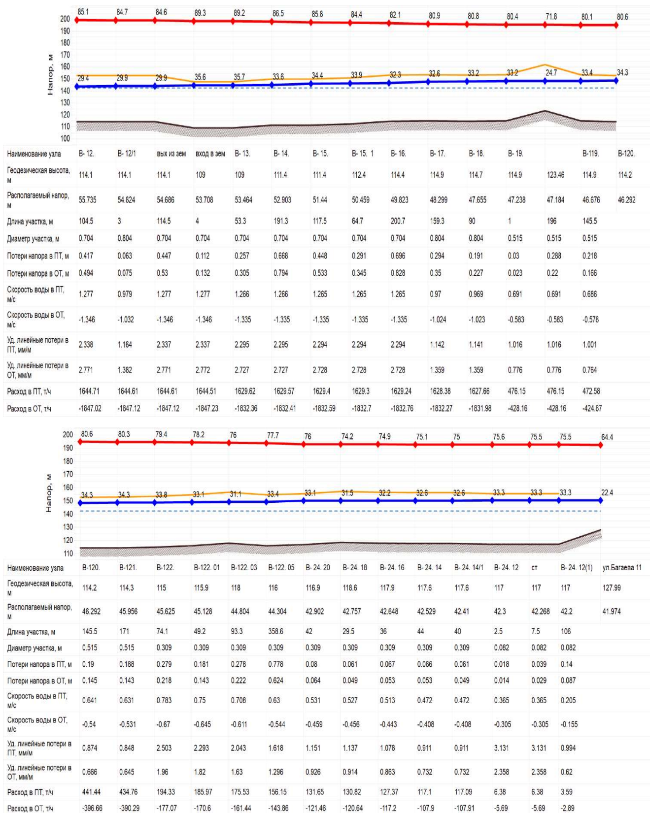
Рисунок 12.1.3.2 Параметры работы теплосети от ИвТЭЦ-2 (вывод С) до ж/д по ул. Багаева, д.11
