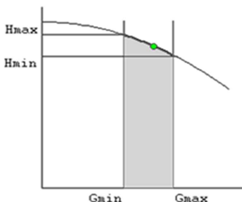
Рисунок 2.5.12 Напорно-расходная характеристика насоса
