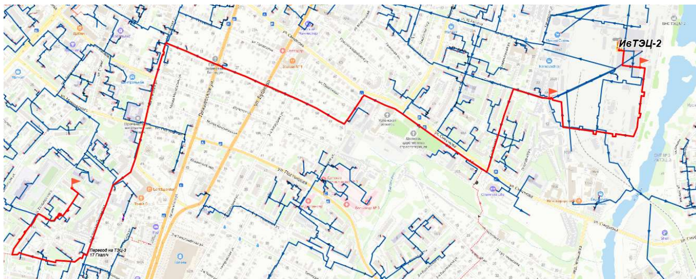
Рисунок 12.1.2.1 Расчетная схема участка теплосети от ИвТЭЦ-2 (вывод В) до ж/д по ул. Володарского, д.7
