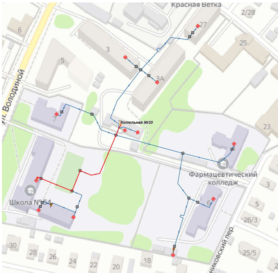
Рисунок 12.2.4.1 Расчетная схема участка теплосети от от Котельной №30 до ж/д №9 по ул. Володиной
