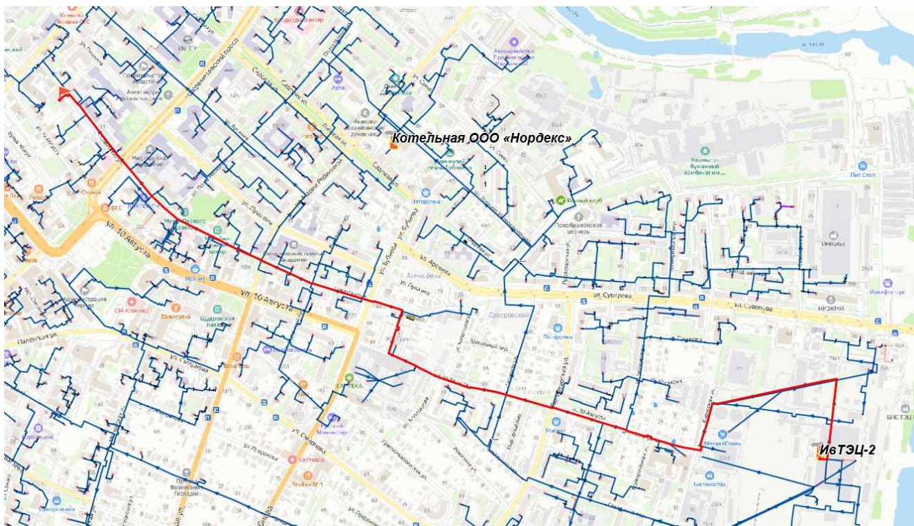
Рисунок 12.1.1.1 Расчетная схема участка теплосети от ИвТЭЦ-2 (вывод А) до ж/д по ул. Советская, д.6
