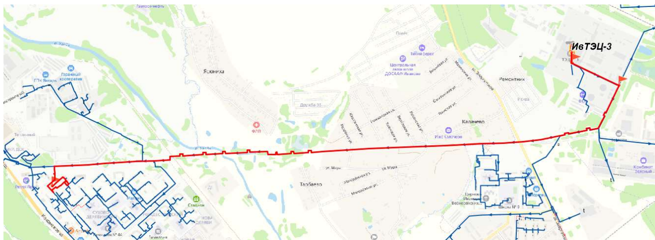
Рисунок 12.1.3.1 Расчетная схема участка теплосети от ИвТЭЦ-3 (вывод D) до ж/д по Кохомскому ш., д.9
