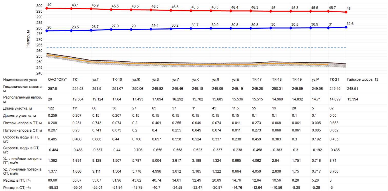
Рисунок 12.2.11.2 Параметры работы теплосети от Котельной №46 до ж/д №4а по ул. Суздальская
