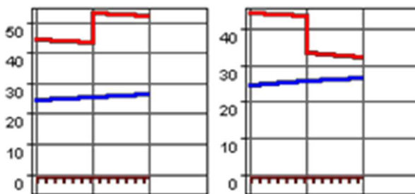
Рисунок 2.5.11 Пьезометрические графики
