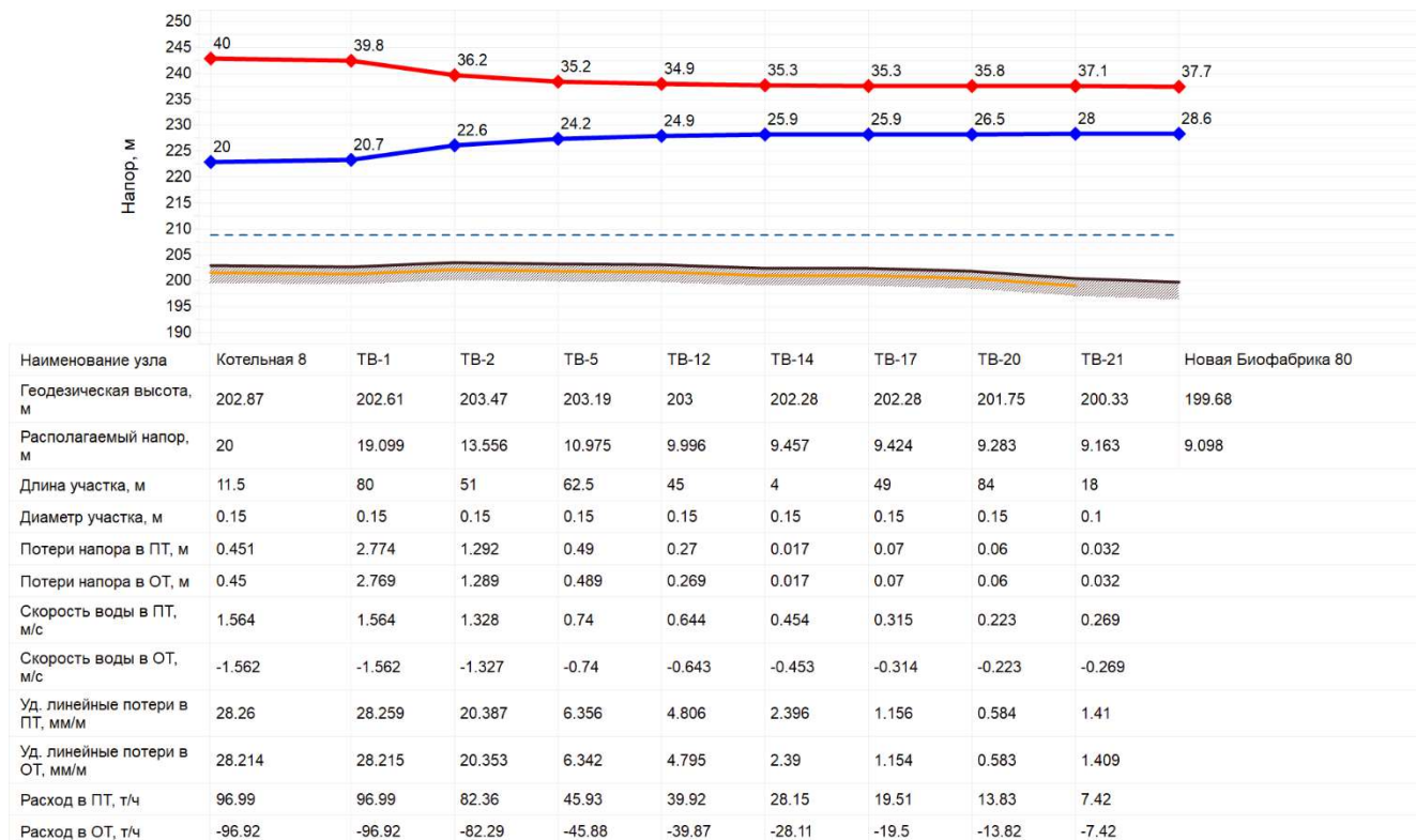
Рисунок 12.2.7.2 Параметры работы теплосети от Котельной №41 до здания по ул. Героя Советского Союза Саха
