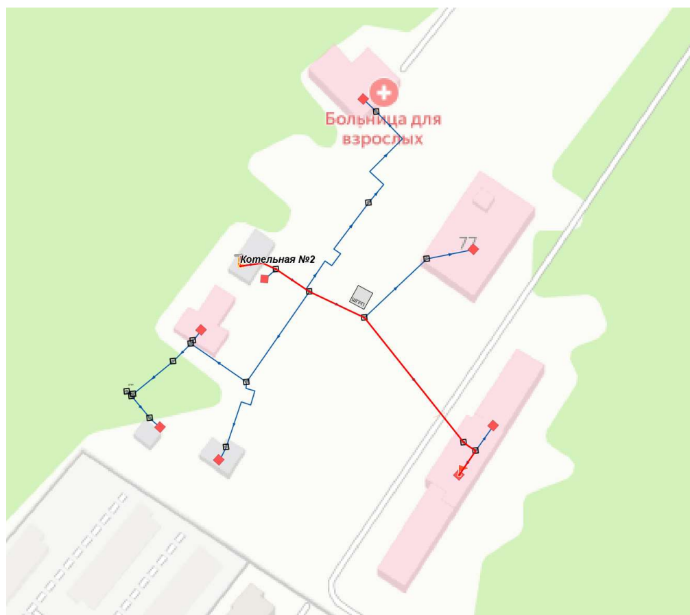
Рисунок 12.2.1.1 Расчетная схема участка теплосети от Котельной №2 до ж/д №77 по ул. Окуловой
