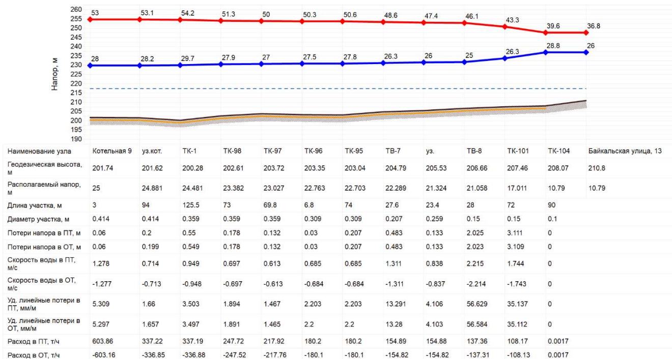
Рисунок 12.2.8.2 Параметры работы теплосети от Котельной №43 до ж/д №1/26 по ул. 9-я линия
