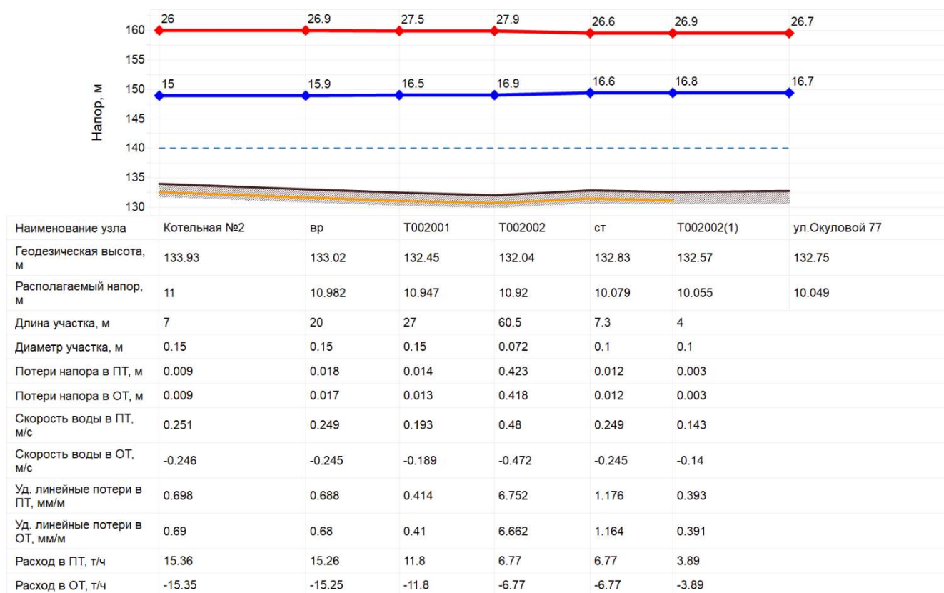
Рисунок 12.2.1.2 Параметры работы теплосети от Котельной №2 до ж/д №77 по ул. Окуловой
