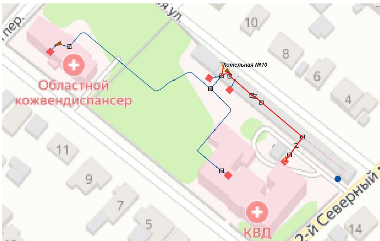
Рисунок 12.2.2.1 Расчетная схема участка теплосети от Котельной №10 до ж/д №2/7 по ул. Детская
