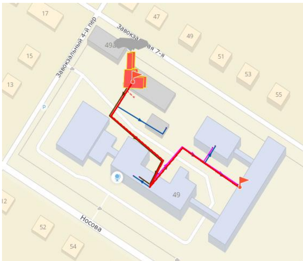
Рис. 5.15 Путь движения теплоносителя от источника тепловой энергии до конечного потребителя, в зоне действия котельной №24
