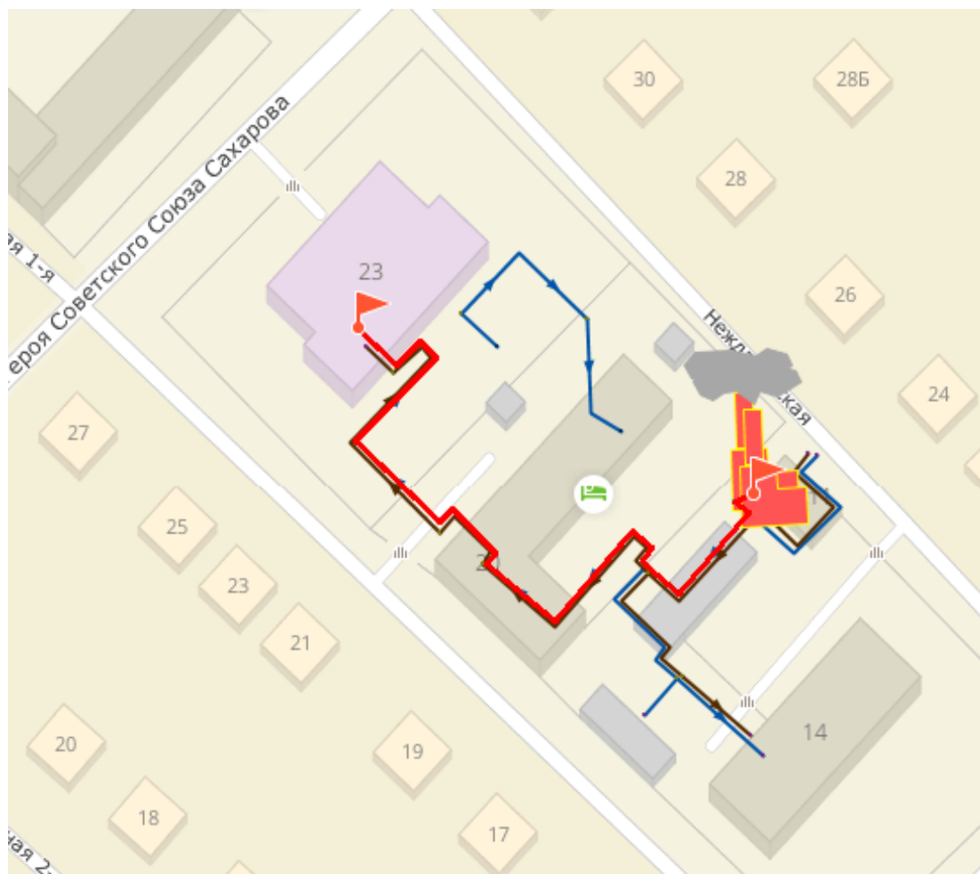
Рис. 5.17 Путь движения теплоносителя от источника тепловой энергии до конечного потребителя, в зоне действия котельной №25
