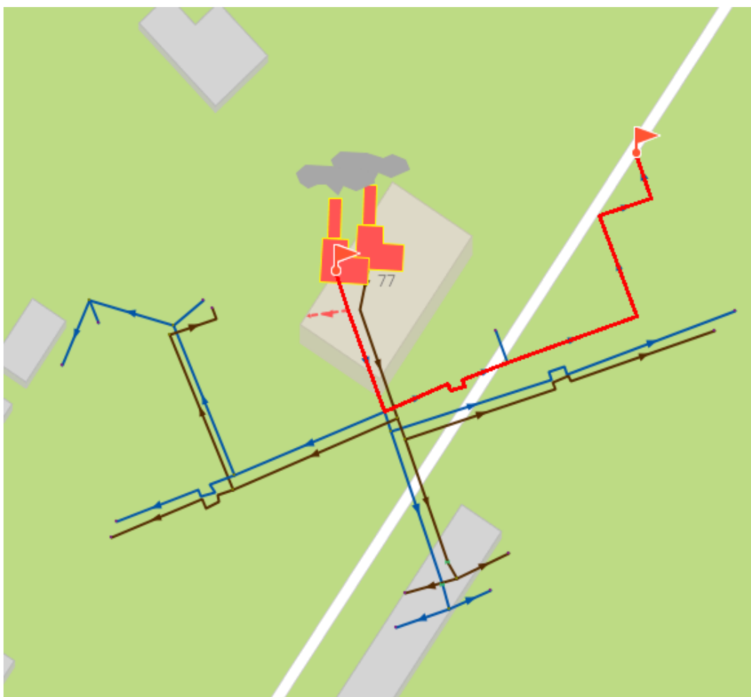
Рис. 5.7 Путь движения теплоносителя от источника тепловой энергии до конечного потребителя, в зоне действия котельной №2
