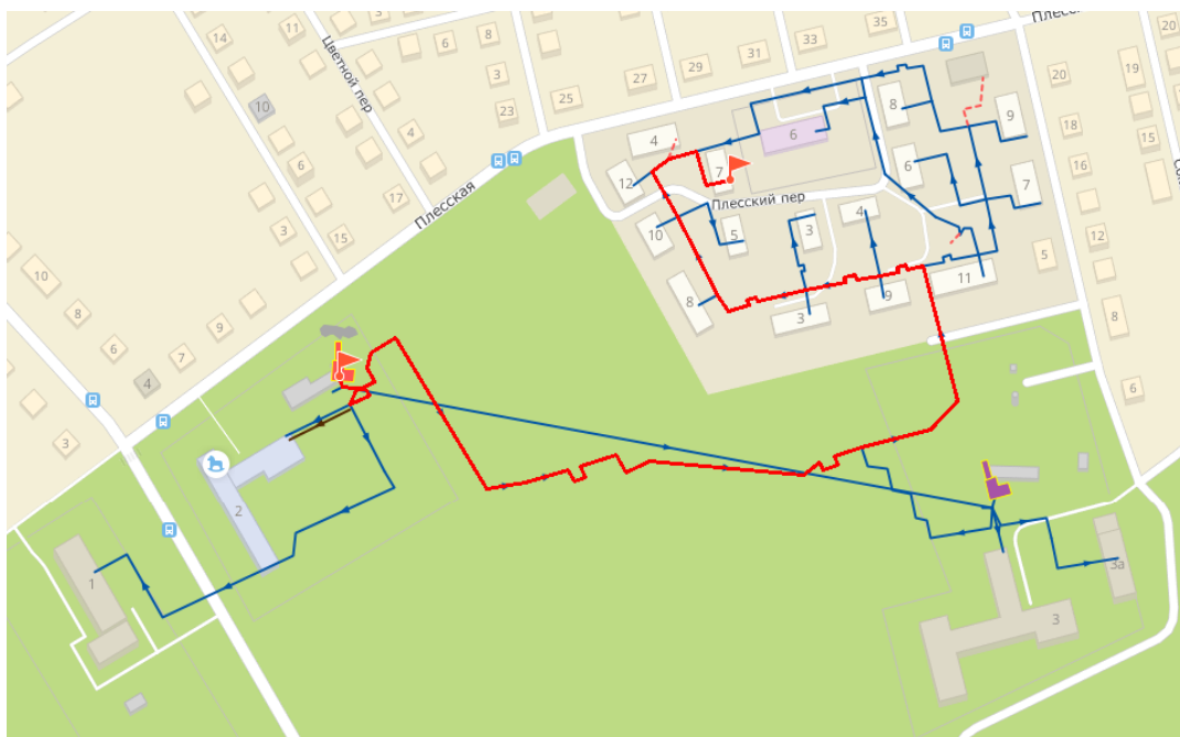
Рис. 5.9 Путь движения теплоносителя от источника тепловой энергии до конечного потребителя, в зоне действия котельной №3
