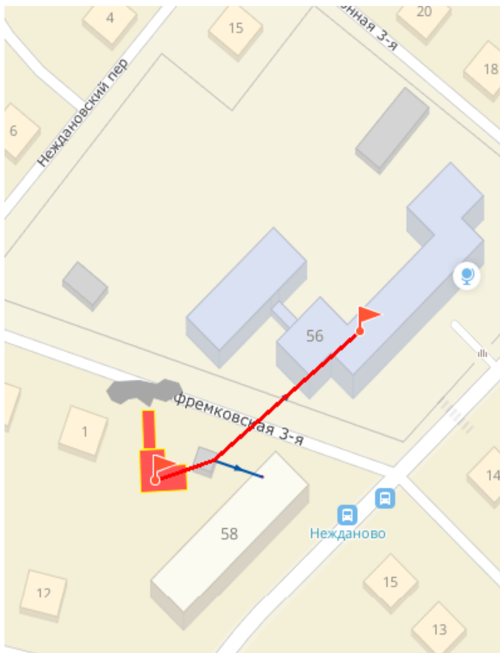
Рис. 5.25 Путь движения теплоносителя от источника тепловой энергии до конечного потребителя, в зоне действия котельной №41
