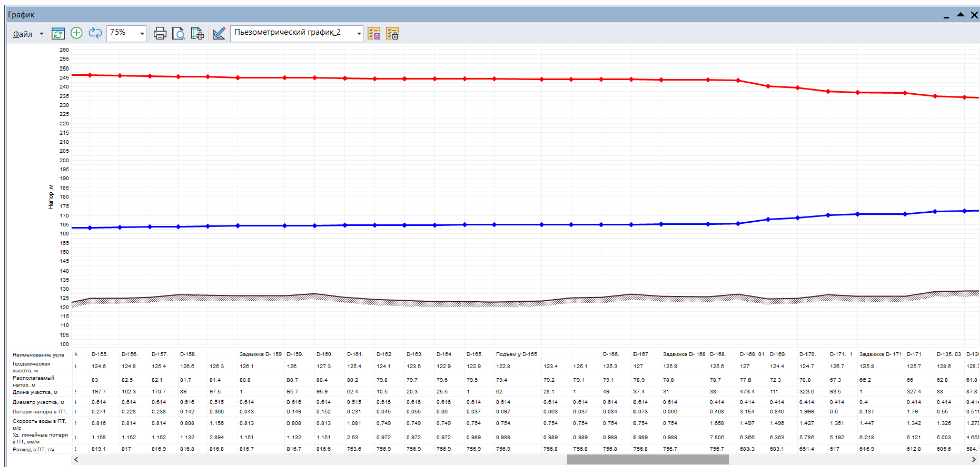
Рис. 13.78 Пьезометрический график от ИвТЭЦ-3 до удаленного потребителя ул.Некрасова 45 (продолжение 3)
