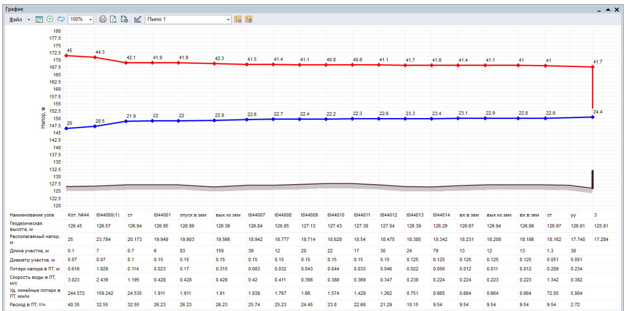
Рис. 13.4 Пьезометрический график от котельной №44 до конечного потребителя
