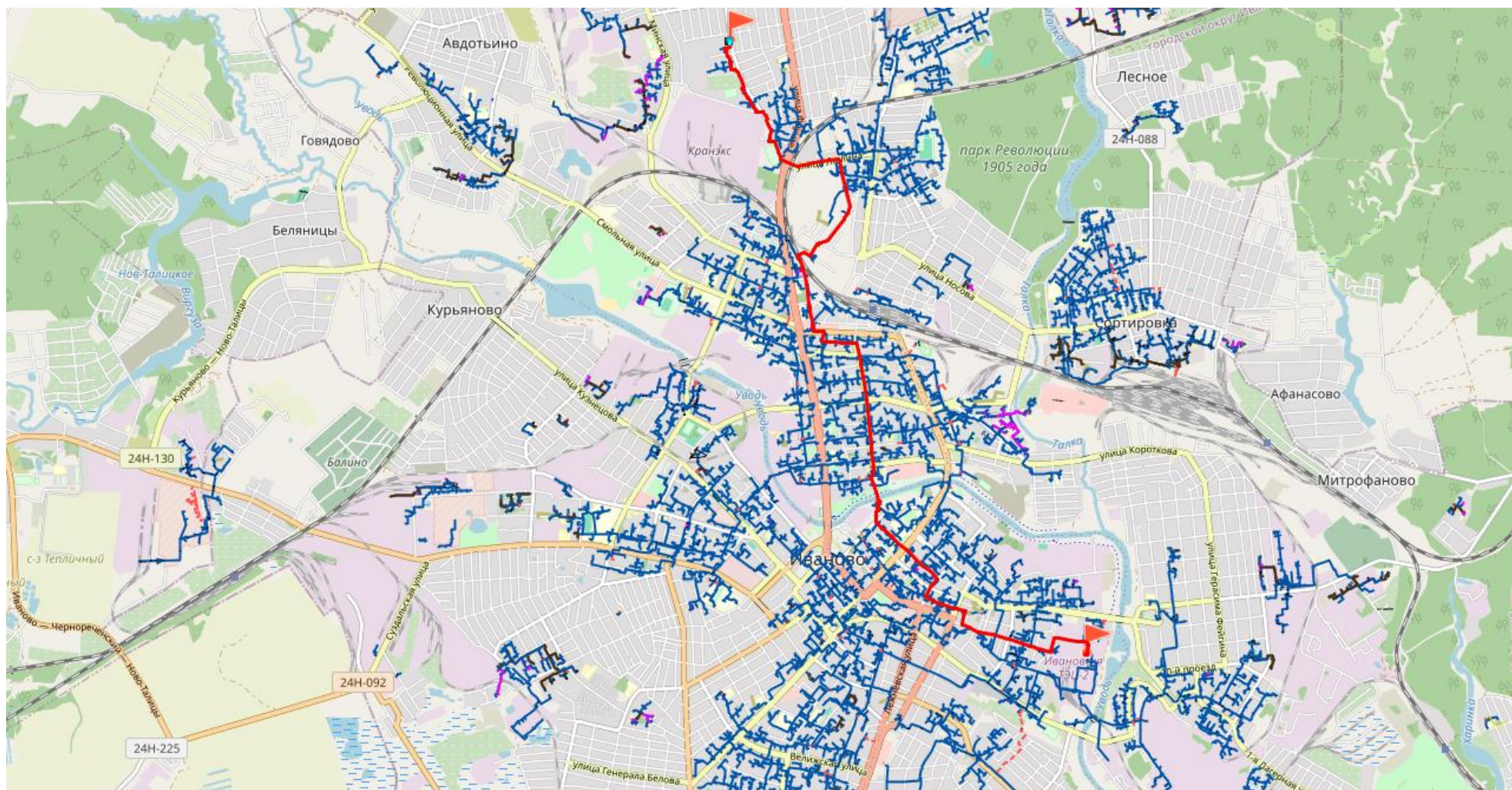
Рис. 13.67 Путь теплоносителя от ИВТЭЦ-2 до удаленного потребителя ул.Генерала Горбатова 19
