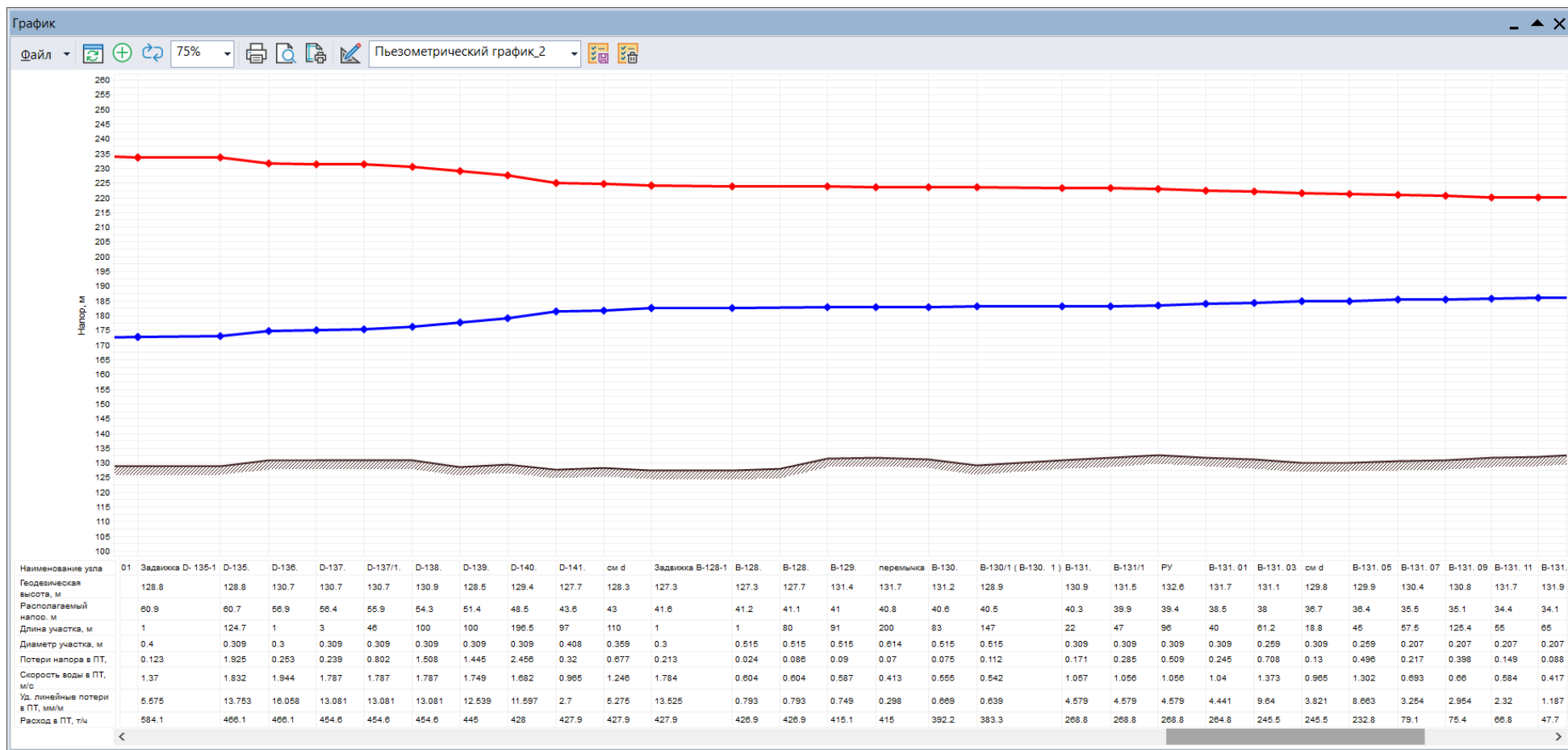
Рис. 13.79 Пьезометрический график от ИвТЭЦ-3 до удаленного потребителя ул.Некрасова 45 (продолжение 4)
