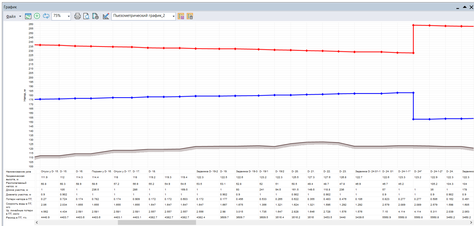
Рис. 13.76 Пьезометрический график от ИвТЭЦ-3 до удаленного потребителя ул.Некрасова 45 (продолжение 1)
