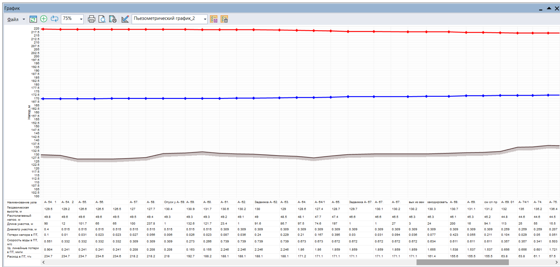
Рис. 13.72 Пьезометрический график от ИвТЭЦ-2 до удаленного потребителя ул.Генерала Горбатова 19 (продолжение 4)
