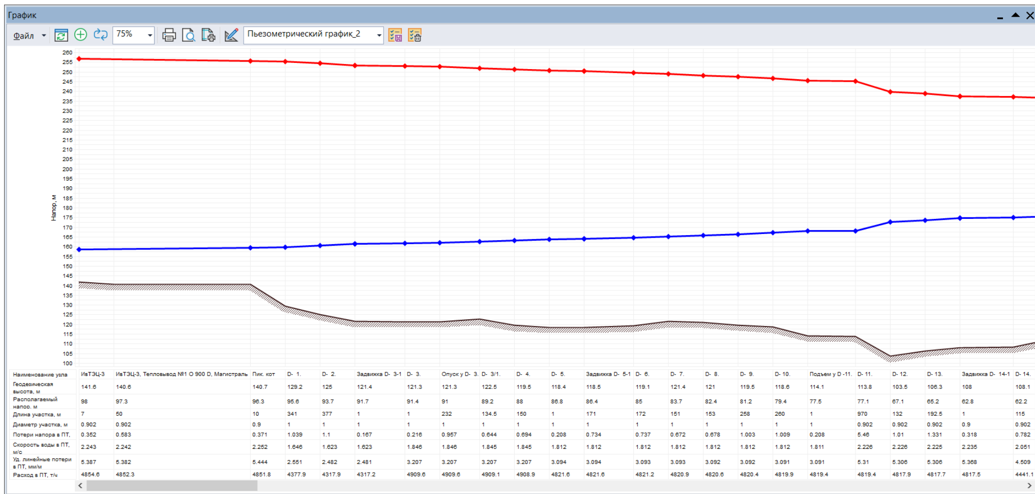
Рис. 13.75 Пьезометрический график от ИвТЭЦ-3 до удаленного потребителя ул.Некрасова 45 (начало)
