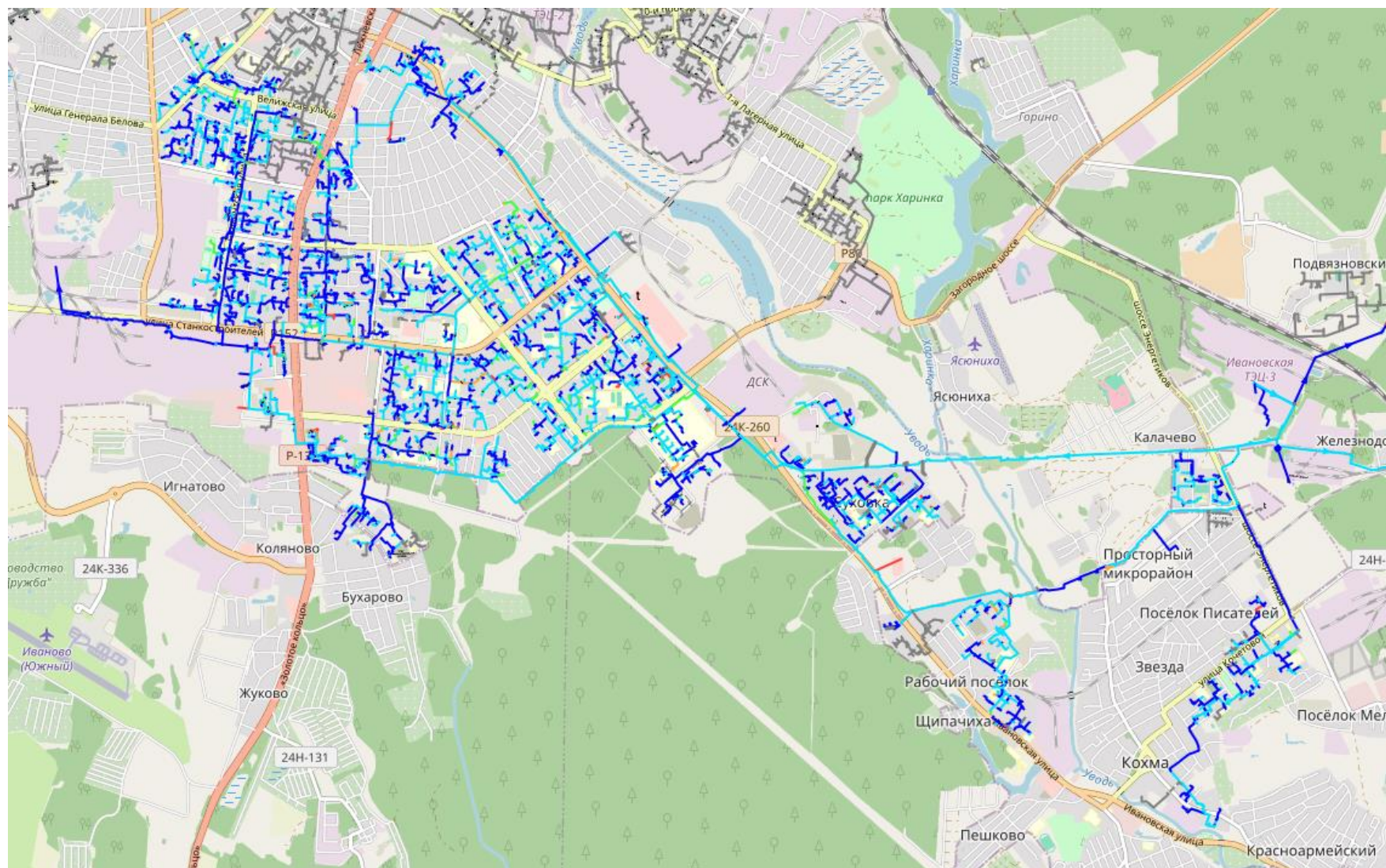
Рис. 13.82 Распределение удельных линейных потерь напора в сетях ИвТЭЦ-3
