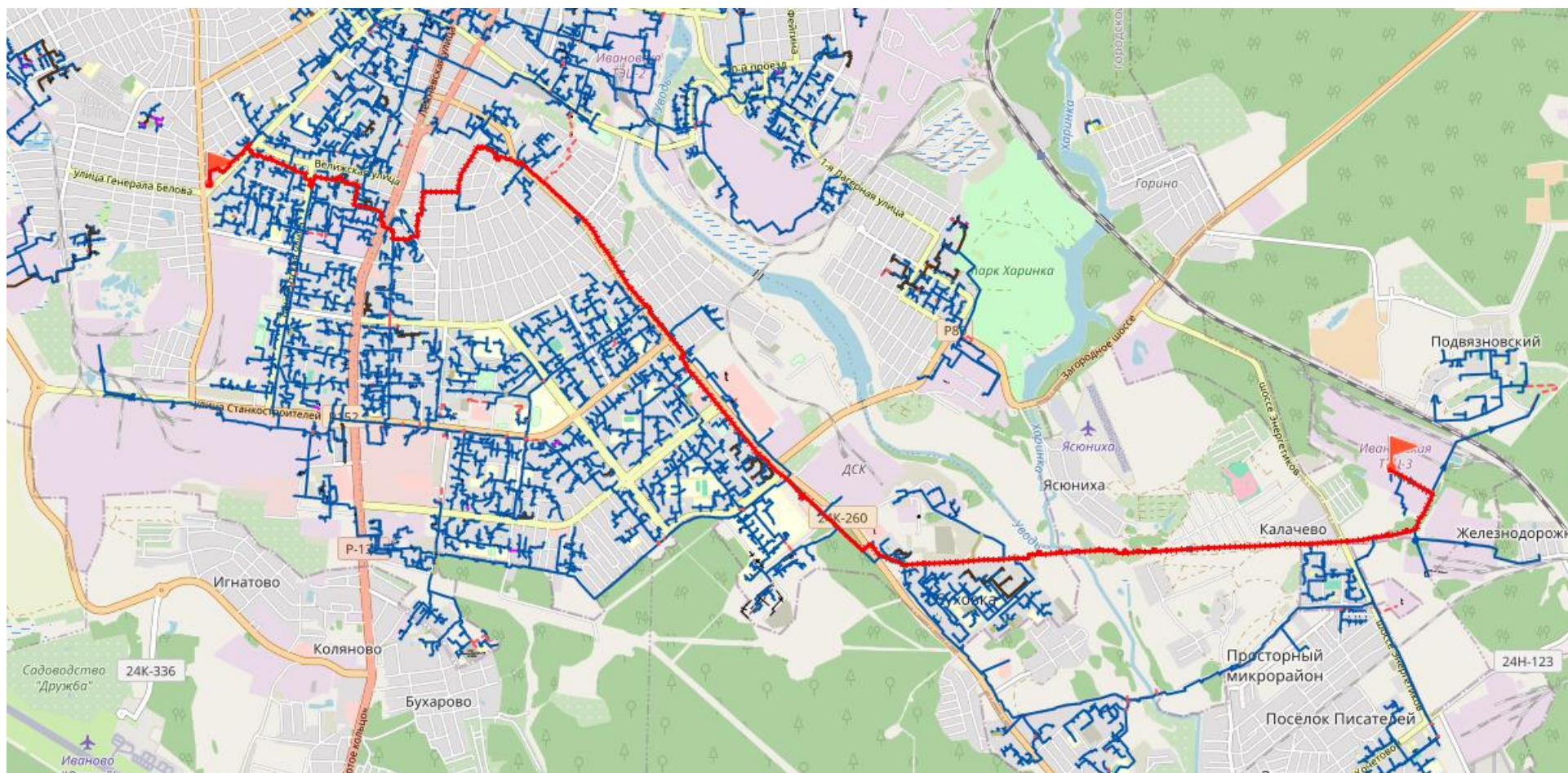
Рис. 13.74 Путь теплоносителя от ИВТЭЦ-3 до удаленного потребителя ул.Некрасова 45
