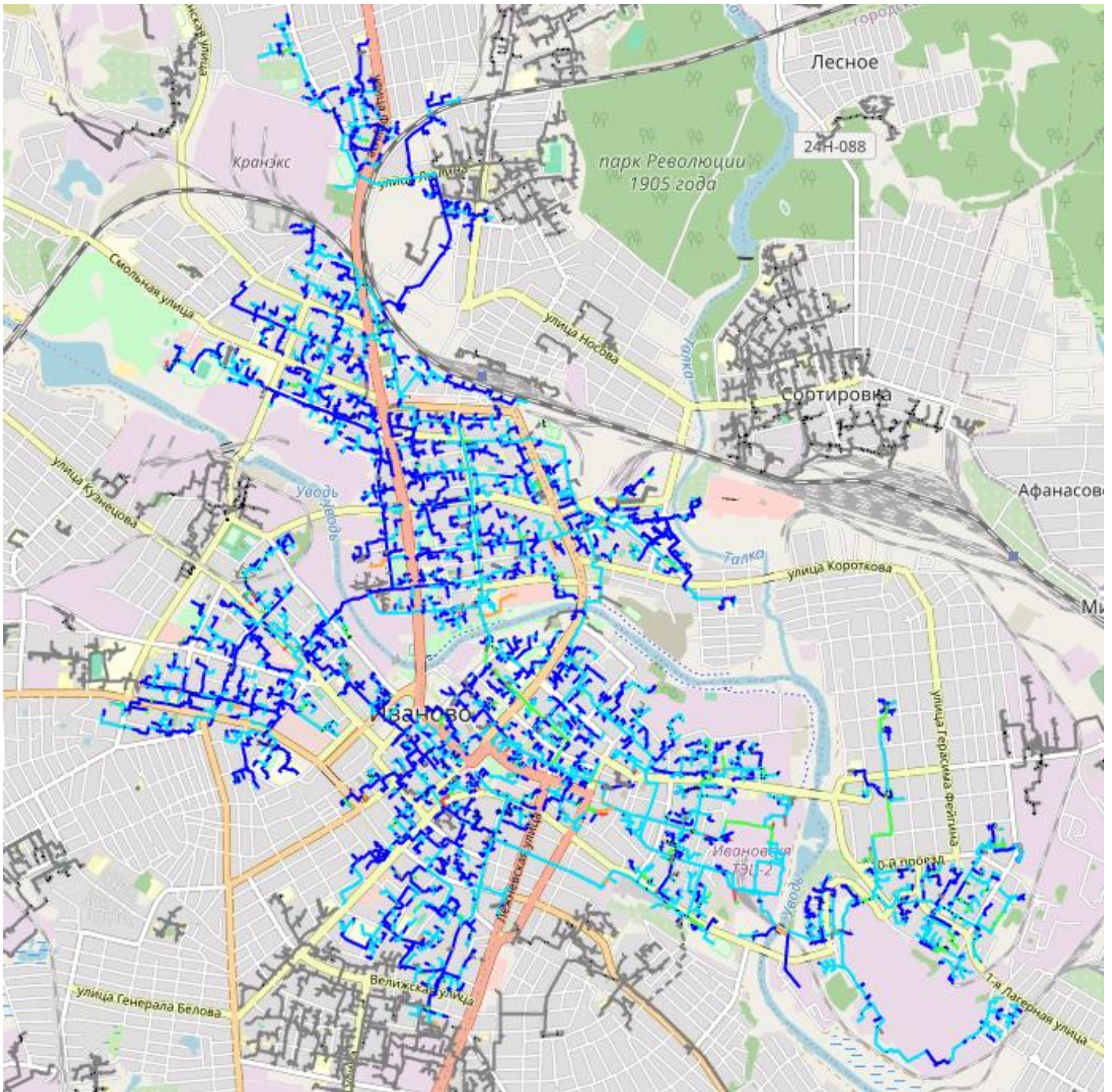
Рис. 13.81 Распределение удельных линейных потерь напора в сетях ИвТЭЦ-2
