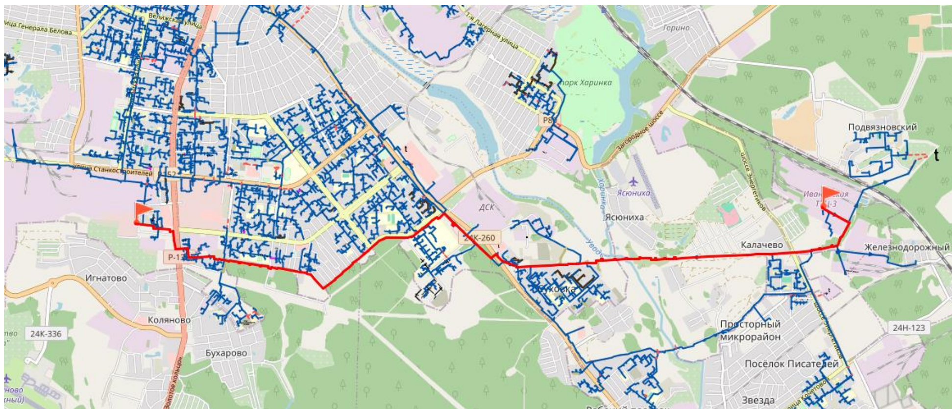
Рис. 13.54 Путь теплоносителя от ИвТЭЦ-3 (вывод E) до удаленного потребителя ул Станкостроителей, 1 стр 2
