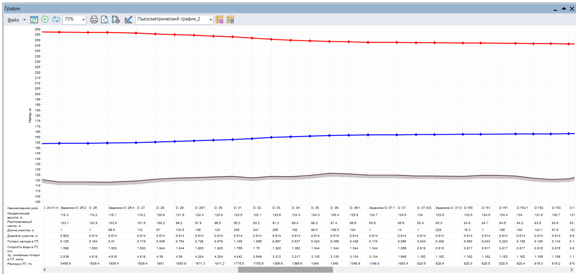
Рис. 13.77 Пьезометрический график от ИвТЭЦ-3 до удаленного потребителя ул.Некрасова 45 (продолжение 2)
