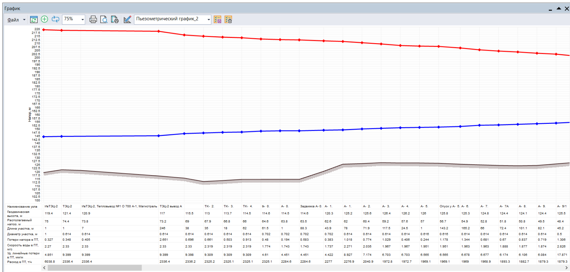
Рис. 13.68 Пьезометрический график от ИвТЭЦ-2 до удаленного потребителя ул.Генерала Горбатова 19 (начало)
