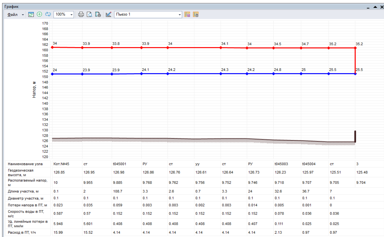
Рис. 13.21 Пьезометрический график от котельной №45 до конечного потребителя
