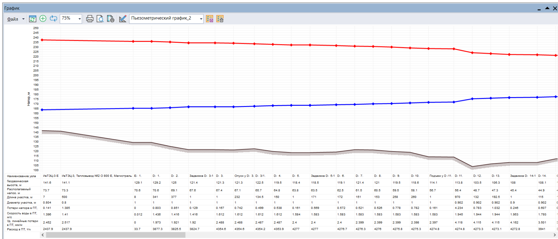
Рис. 13.55 Пьезометрический график от ИвТЭЦ-3 (вывод Е) до удаленного потребителя ул Станкостроителей, 1 стр 2 (начало)
