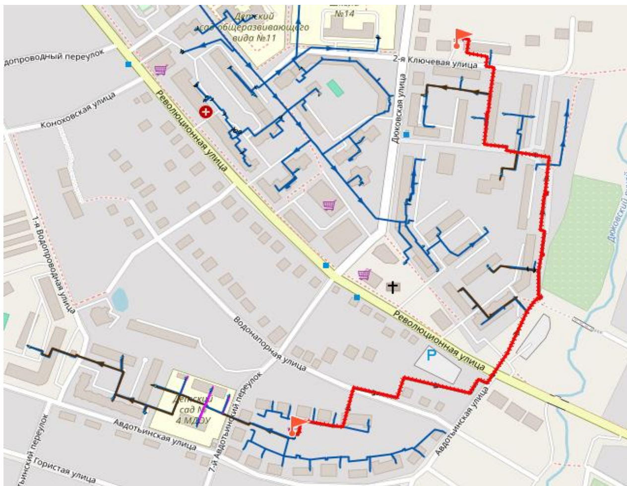
Рис. 13.37 Путь теплоносителя от котельной №33 до конечного потребителя
