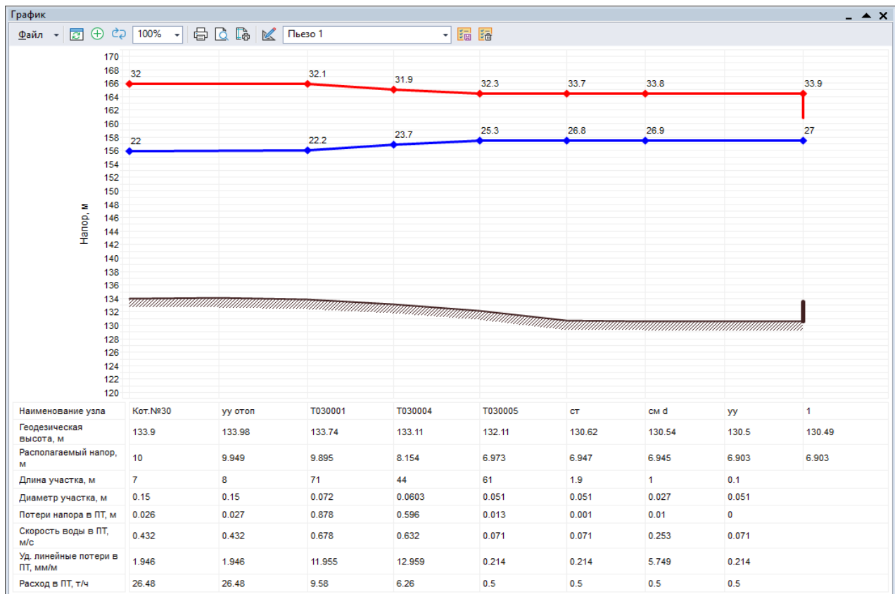
Рис. 13.10 Пьезометрический график от котельной №30 до конечного потребителя
