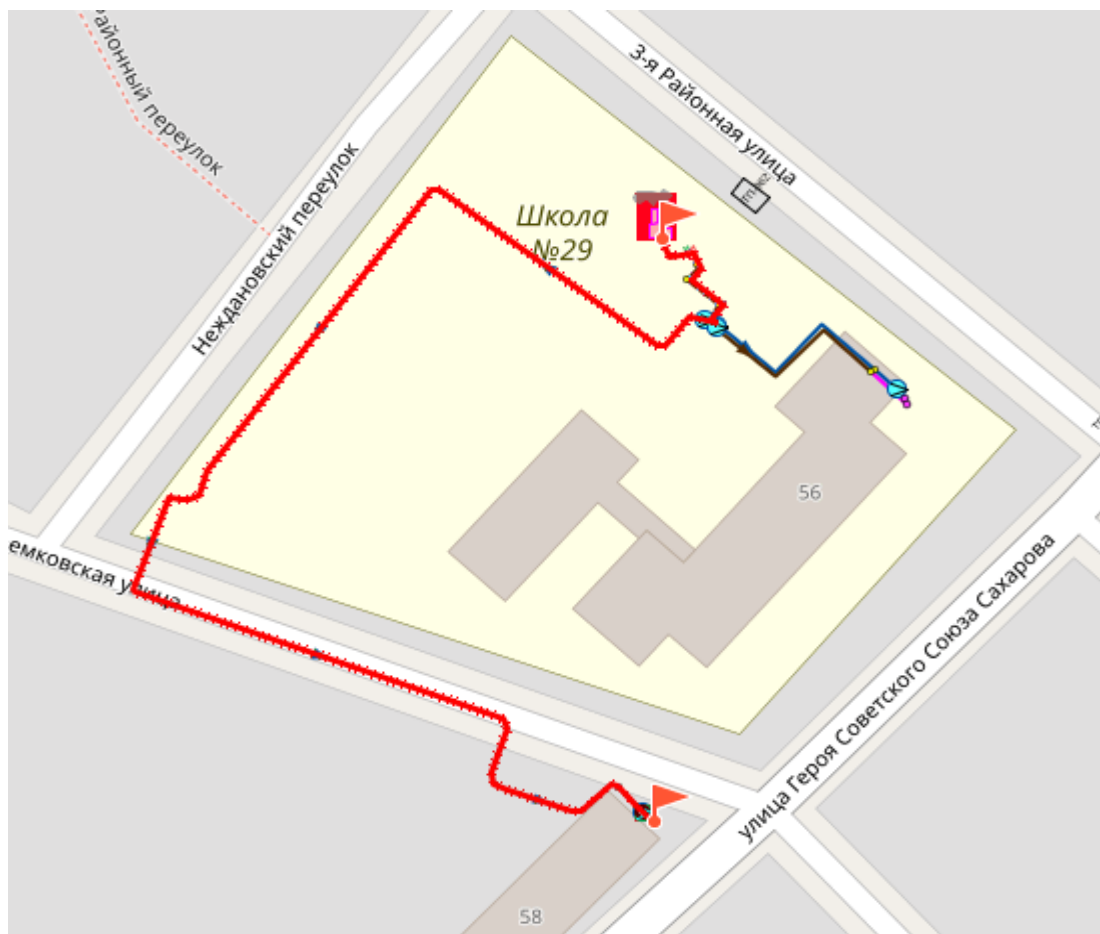
Рис. 13.16 Путь теплоносителя от котельной №41 до конечного потребителя
