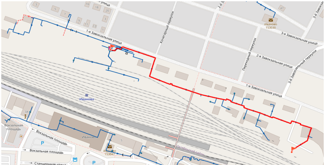
Рис. 13.3 Путь теплоносителя от котельной №44 до конечного потребителя
