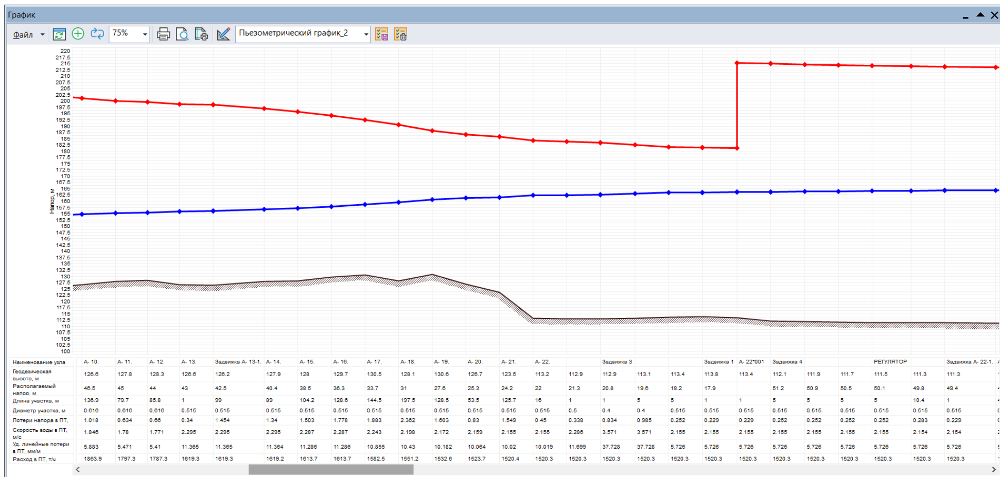
Рис. 13.69 Пьезометрический график от ИвТЭЦ-2 до удаленного потребителя ул.Генерала Горбатова 19 (продолжение 1)
