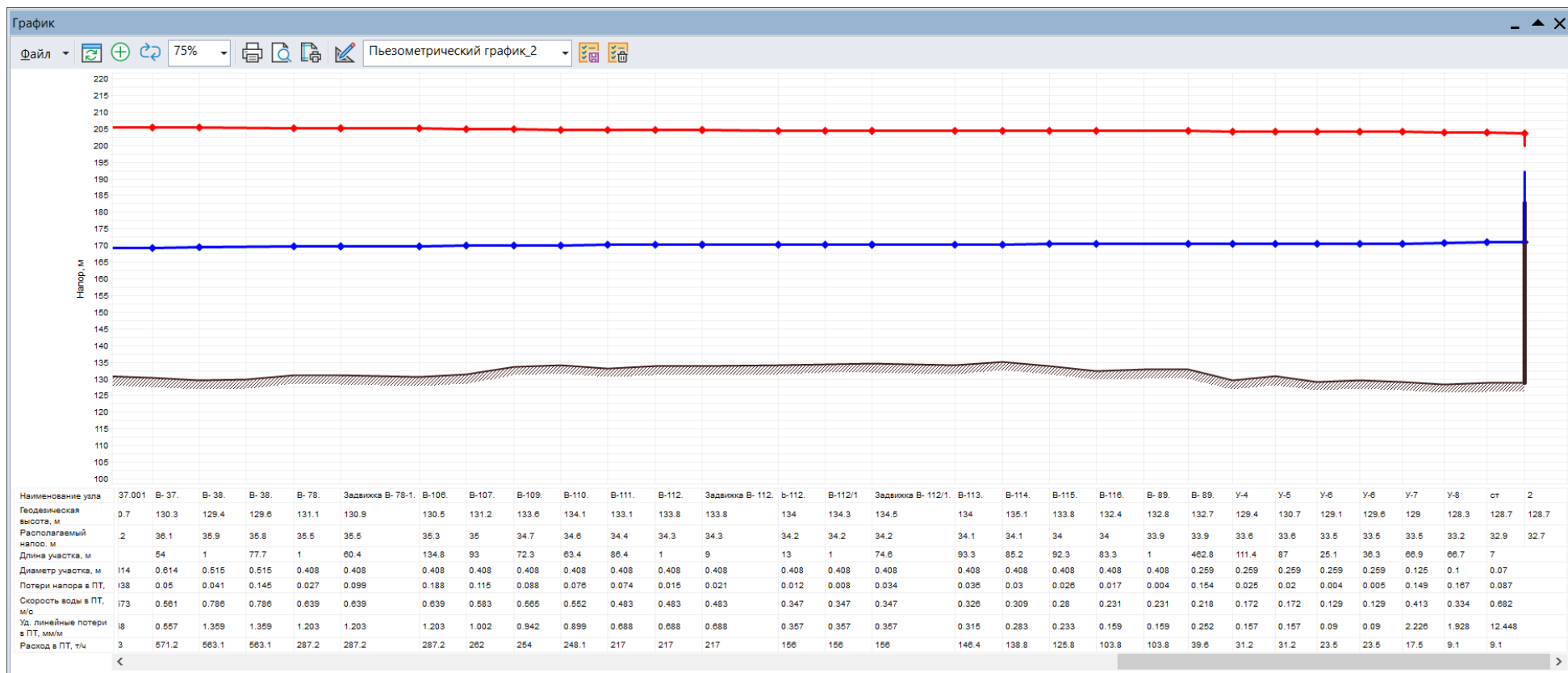
Рис. 13.50 Пьезометрический график от ИвТЭЦ-2 (вывод В) до удаленного потребителя ул.Парижской Коммуны 41 (окончание)
