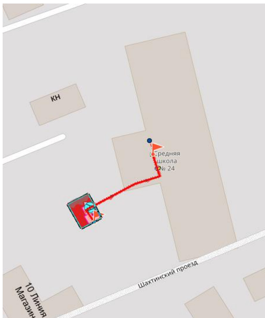
Рис. 13.18 Путь теплоносителя от котельной №43 до конечного потребителя
